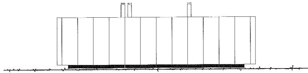
f a s a d - s t ä n g d , skala 1:200
