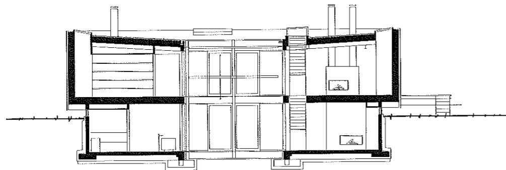
huvudsektion, skala 1:200
