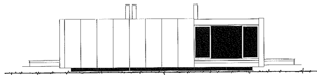
f a s a d - ö p p e n , skala 1:200
