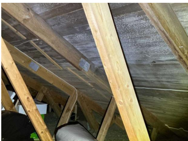
Bild 5: - Utvändigt, Vind, Mikrobiellpäväxt och fuktrosor noteras på underlagstaket
