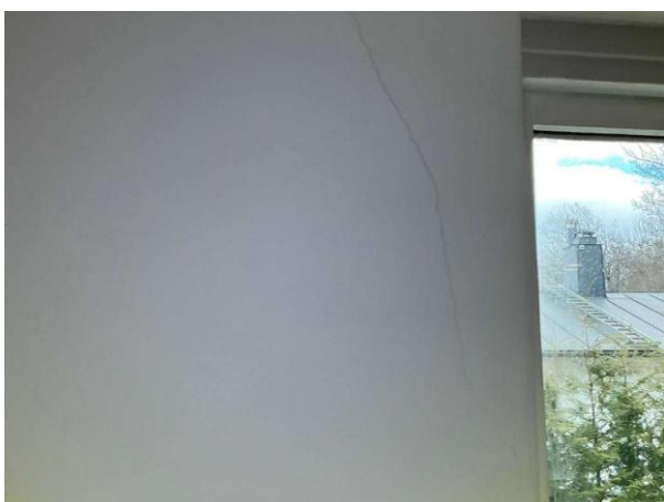
Bild 11: Invändigt, Soutterrängplan, Rörelse sprickor noteras på väggar
