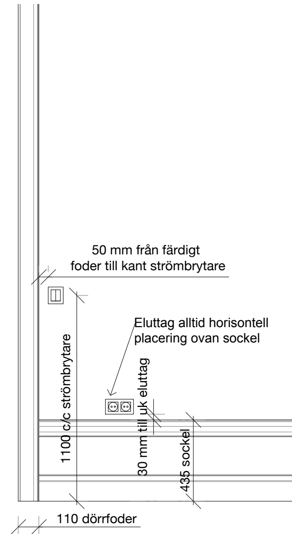
01 PRINCIP FÖR EL PLACERING SKALA 1:20
